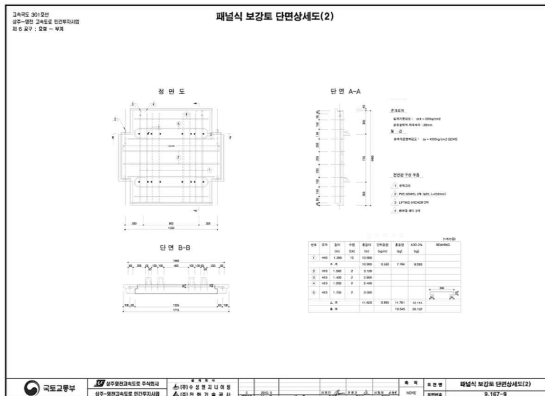
【그림 7.5】 단면도(계속)
