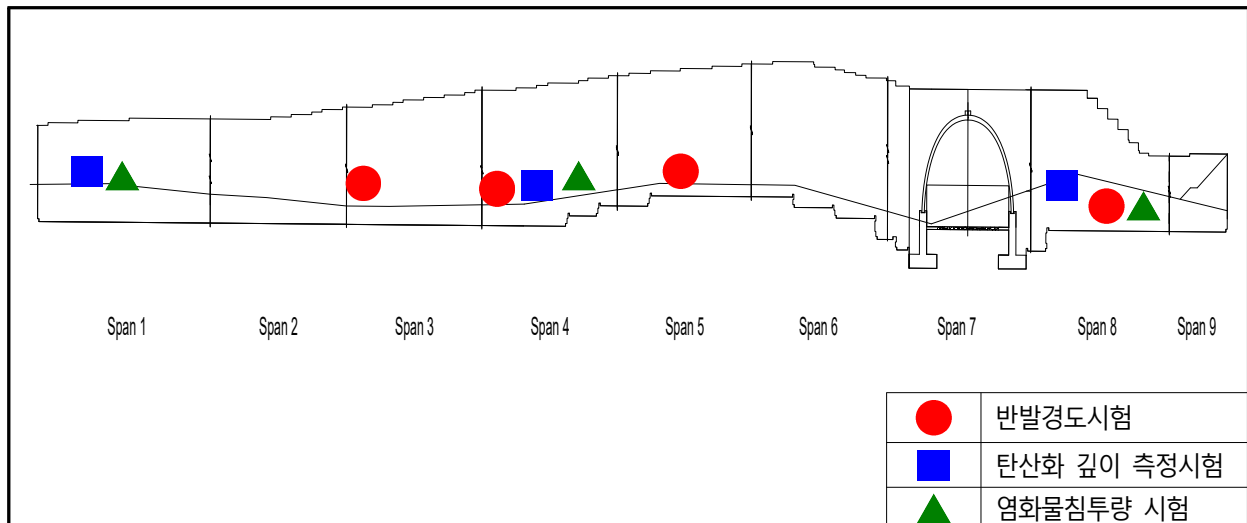
【그림 73.6】 콘크리트 재료시험 조사 위치도
