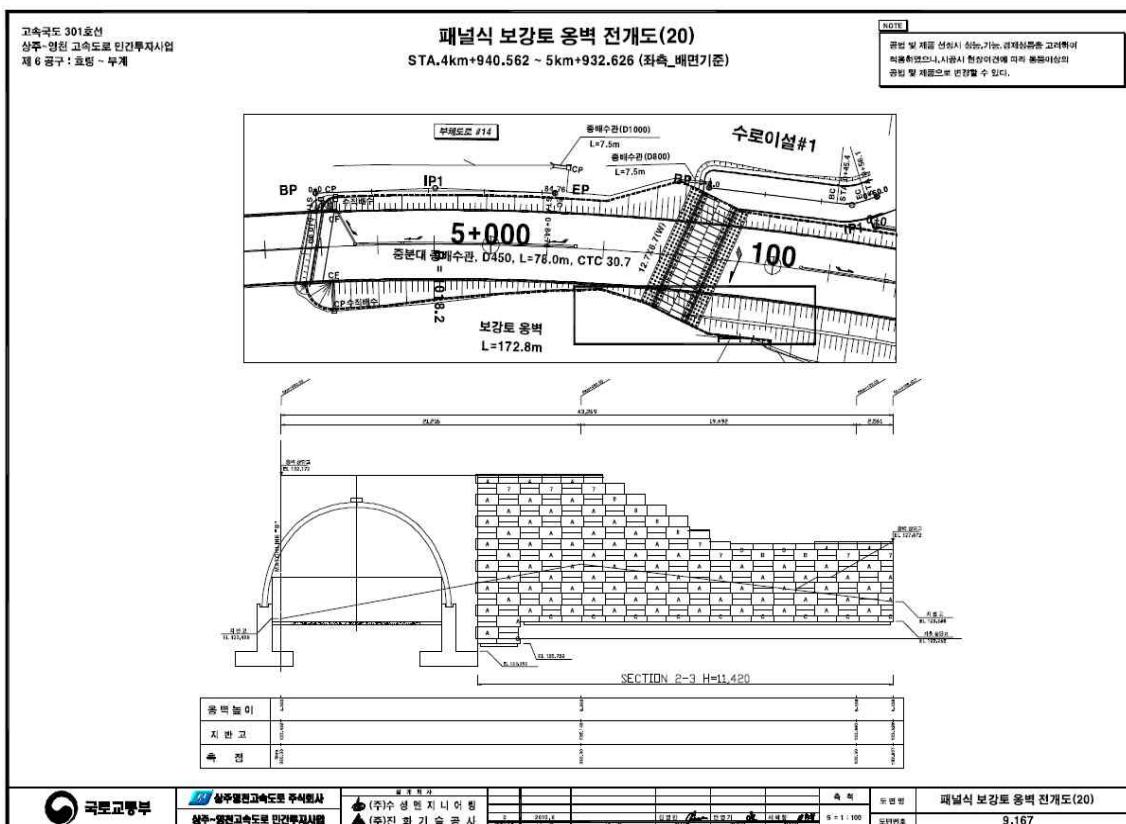
【그림 73.4】전개도
