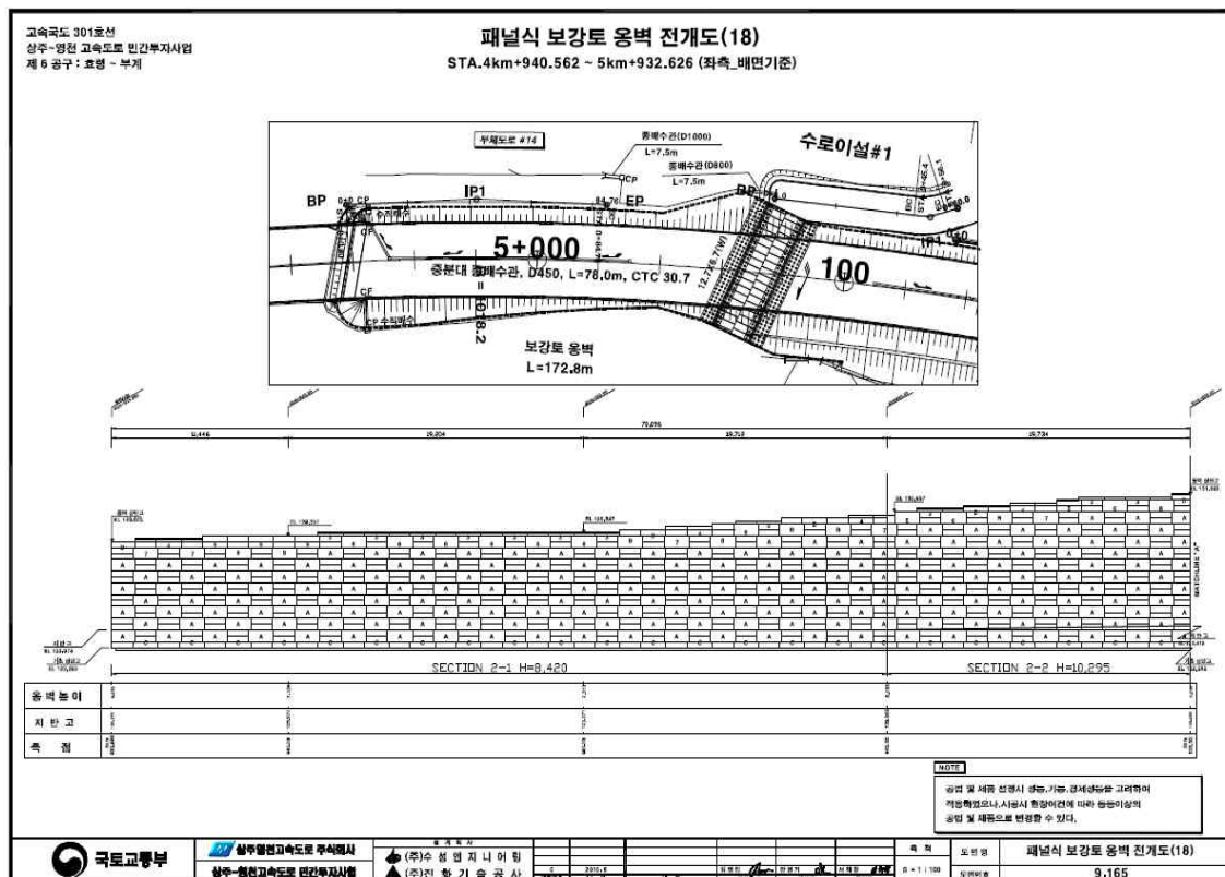
【그림 73.3】 종평면도 및 전개도
