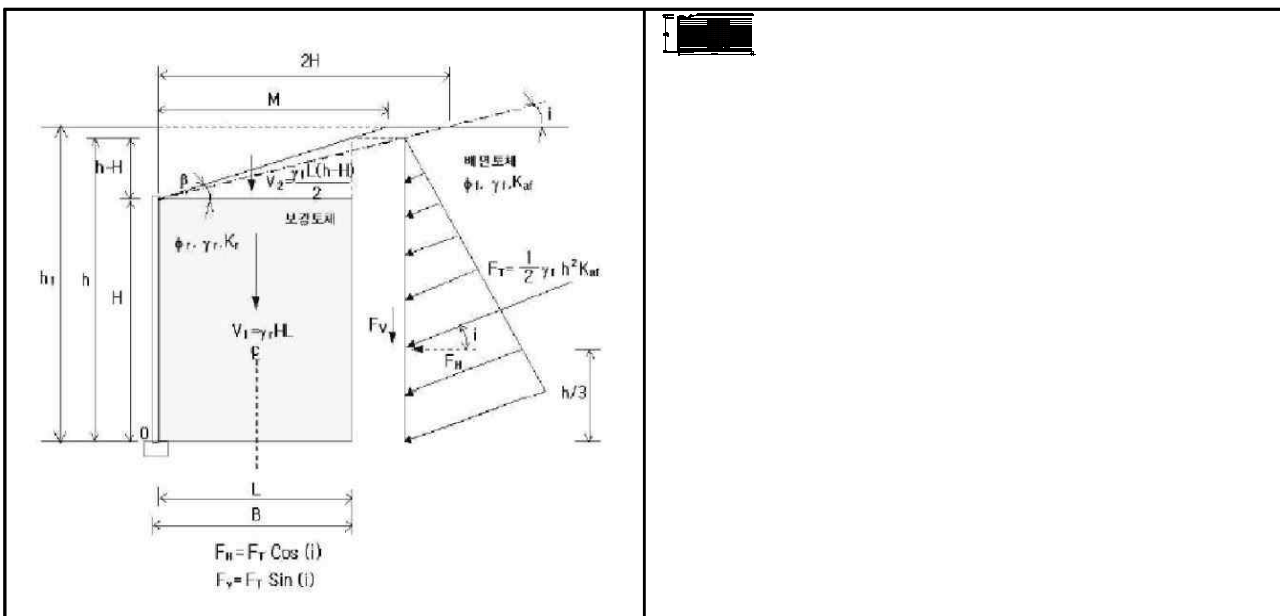
【그림 73.11】 검토단면도
