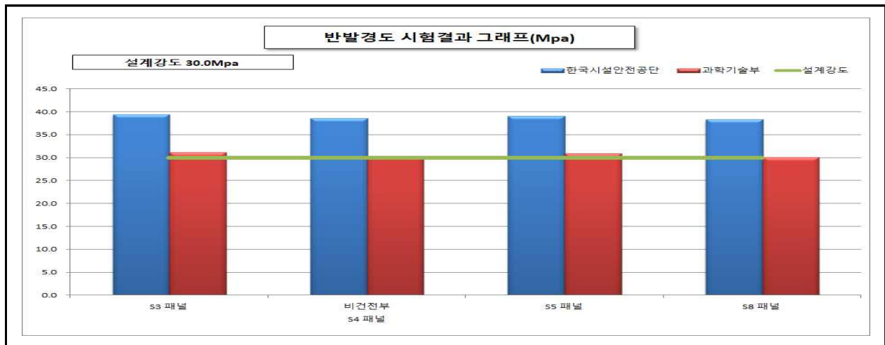
【그림 73.7】 반발경도시험 측정결과
