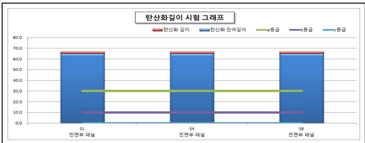
【그림 73.8】 탄산화 깊이 측정결과
